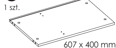
6 Półka prawa
